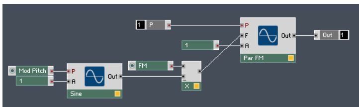
Fig. 6.33 A simple implementation of the Par FM Module.
