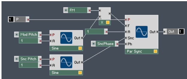
Fig. 6.36 A simple implementation of the Par Sync Module.
